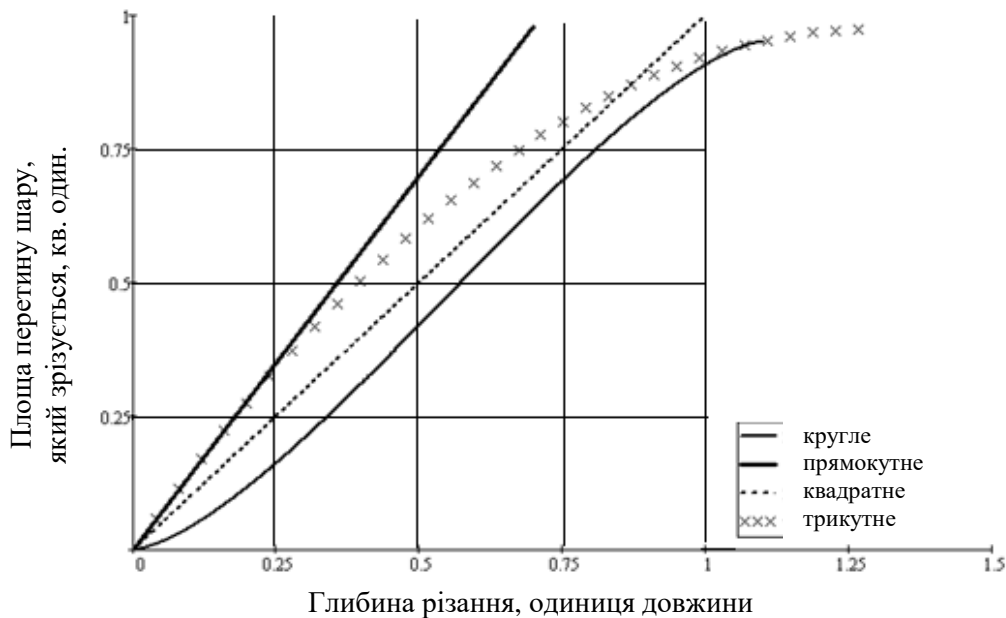
Рисунок 1.2 – Залежності площі перетину зрізаного шару від глибини різання для корпусів різної форми поперечного перетину при одиничному об'ємі і одиничній довжини корпусу
